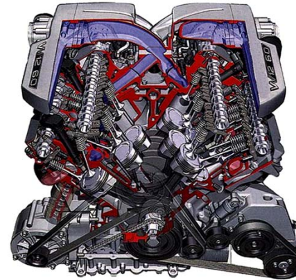
12 cylindres
