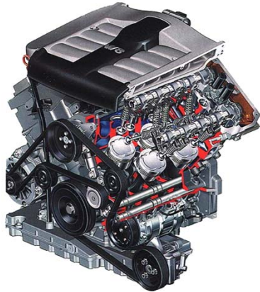
8 cylindres
