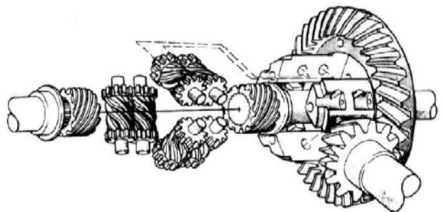
Le différentiel TORSEN
