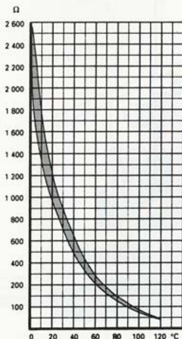
Variation de la résistance du transmetteur en fonction de la température du liquide de refroidissement
