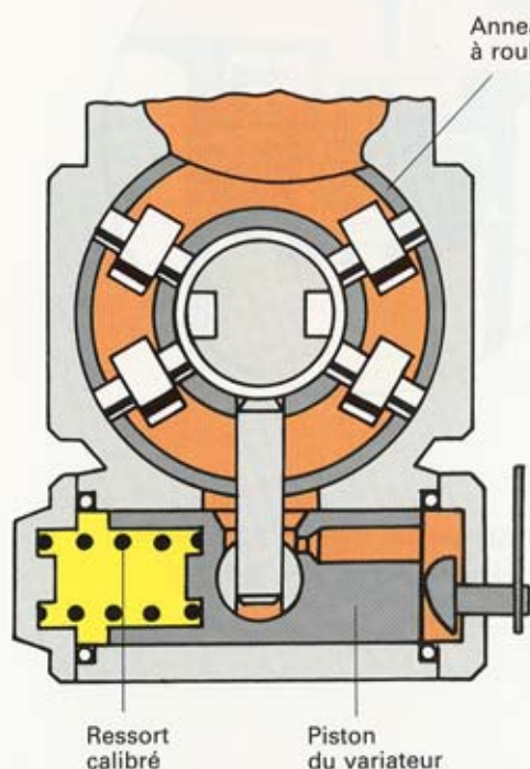
Basse pression dans le corps de la pompe
