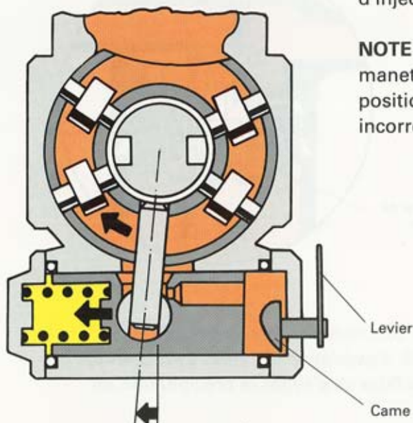
Haute pression dans le corps de la pompe
